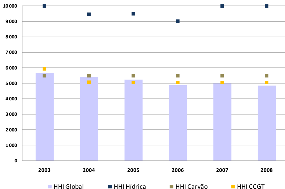
Figura 3-5 - Concentração na produção relativa à capacidade instalada
