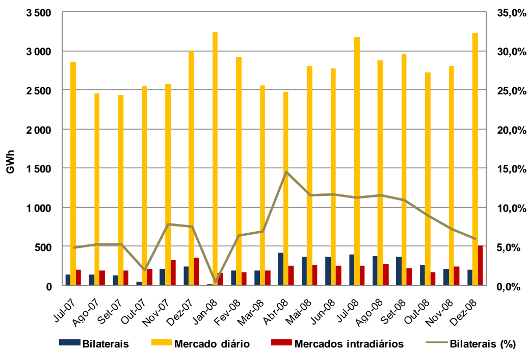
Figura 3-8 – Repartição de volumes de energia entre mercados
