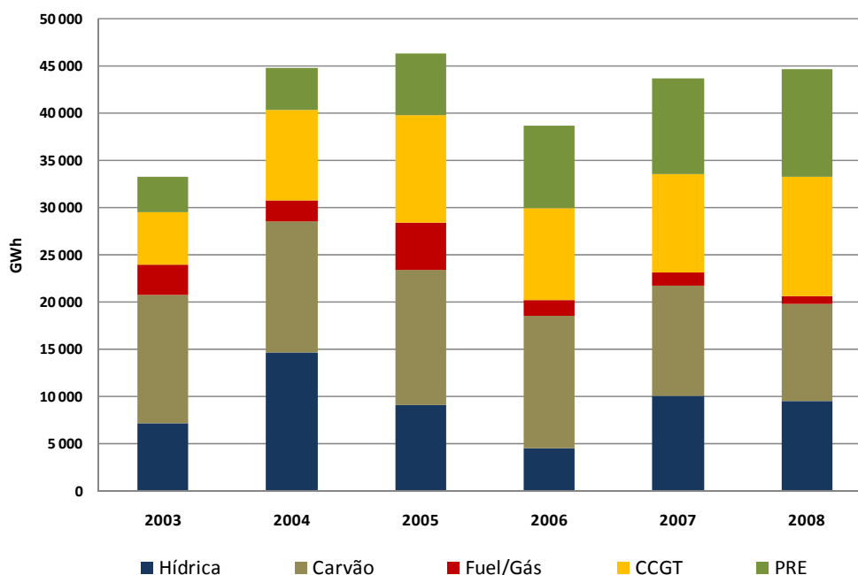
Figura 3-4 - Caracterização do parque electroprodutor em Portugal Por tipo de produção e energia produzida
