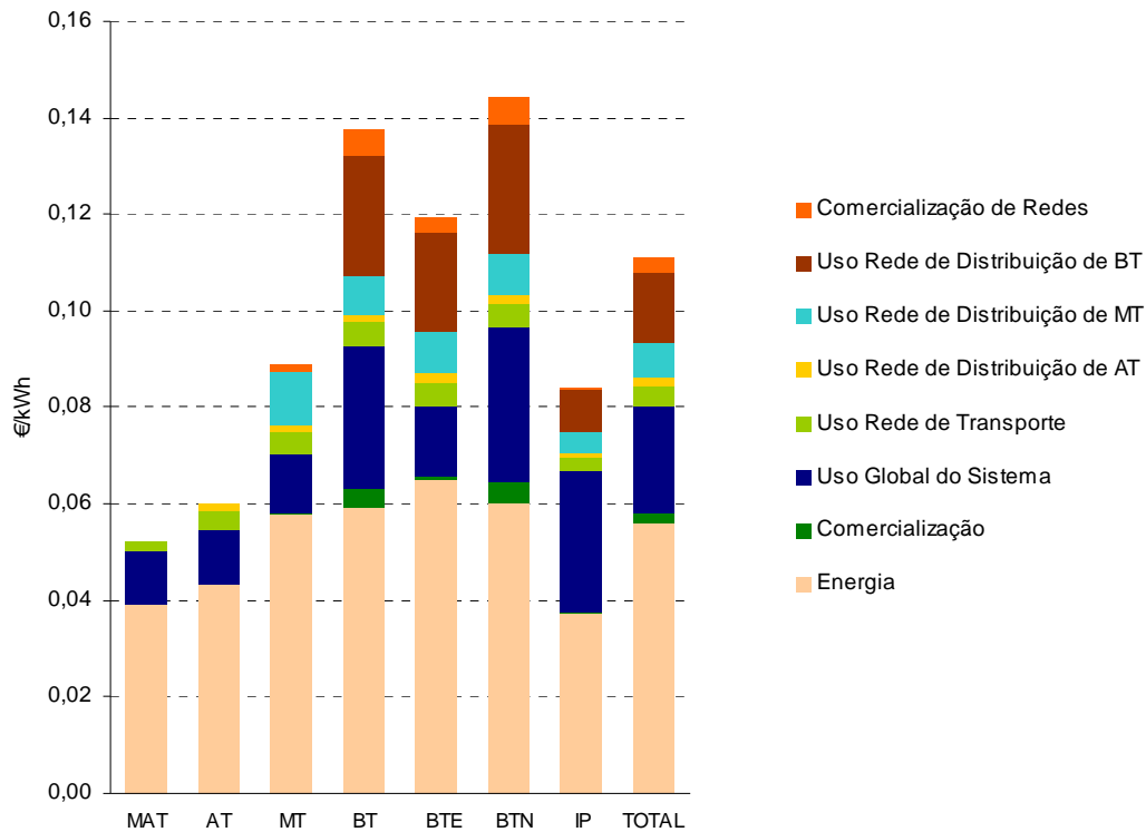
Figura 3-12 – Preço médio das tarifas de Venda a Clientes Finais do comercializador de último recurso em 2008
