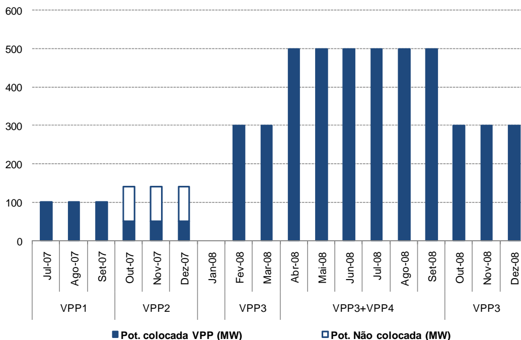
Figura 3-16 – Colocação de capacidade nos leilões VPP
