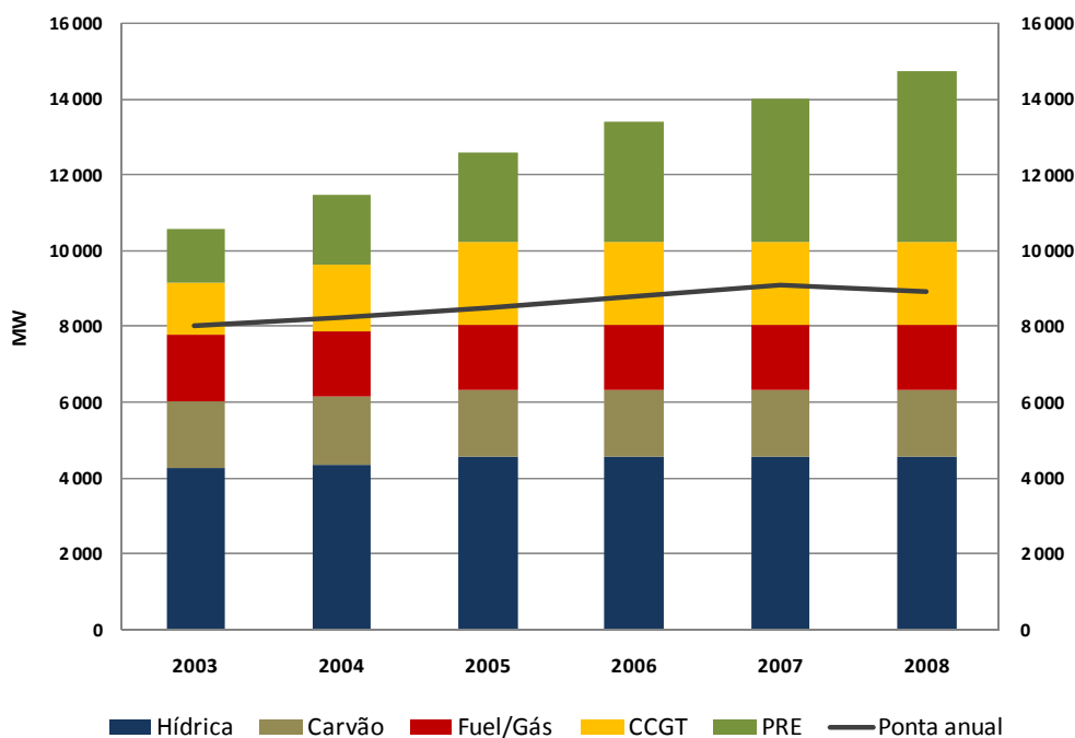
Figura 3-2 - Caracterização do parque electroprodutor em Portugal Por tipo de produção e capacidade instalada
